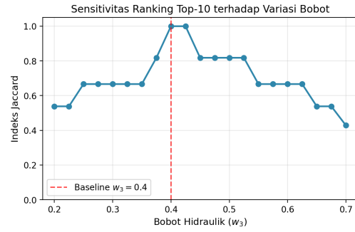
Fig. 2. Analisis Sensitivitas Bobot
